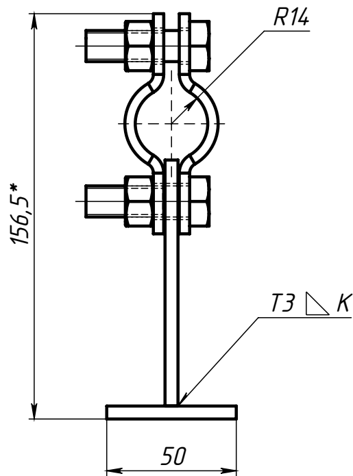
Поз.3 (Полухомут)
