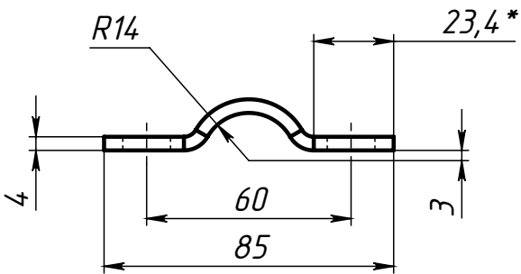
Поз.3 (Полухомут)
