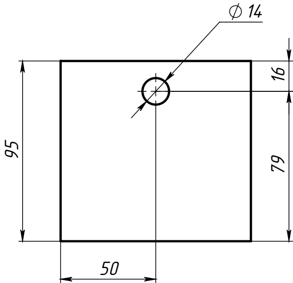
Поз.2 (Ребро)
